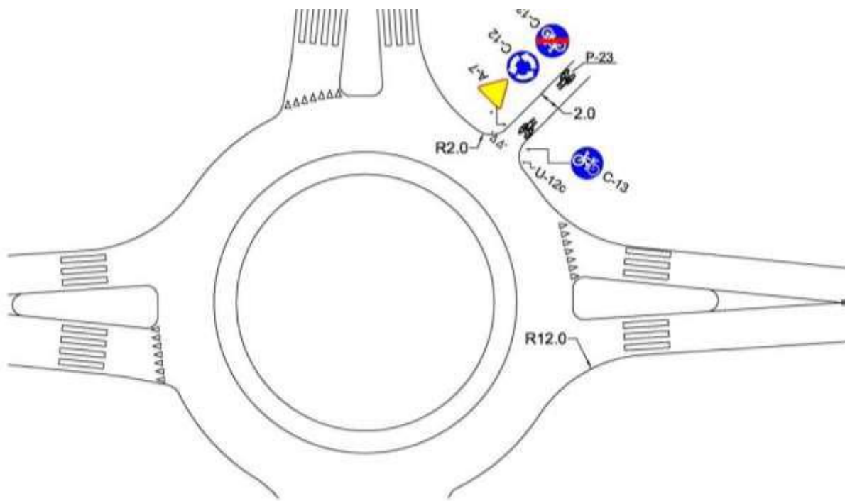
Rysunek 19. Dwukierunkowa trasa rowerowa jako samodzielny wlot jednopasowego małego ronda
