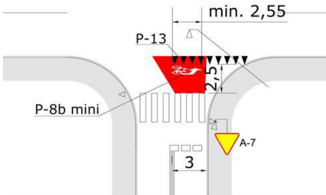
Rysunek 10. Śluza dla rowerów – typu 2
