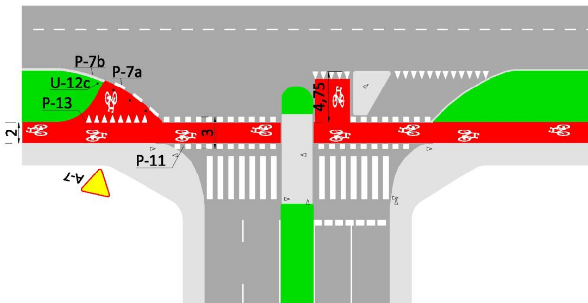
Rysunek 12. Śluzę dla rowerów typu 3 (pośrodku, między przejazdem dla rowerzystów a skrzyżowaniem) oraz typu 4 (po lewej stronie rysunku)
