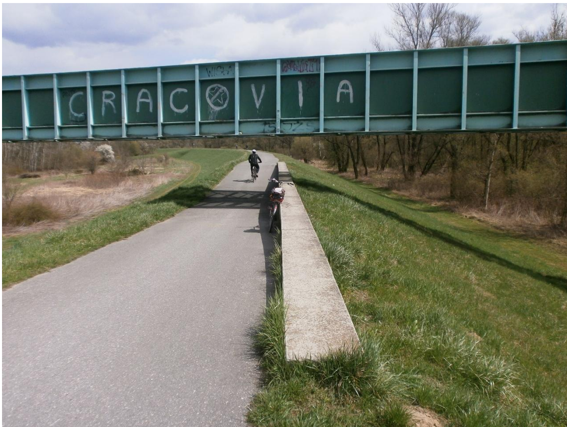
Ilustracja 4. Mur oporowy umożliwiający miejscowe obniżenie niwelety korony wału pod przeszkodą
