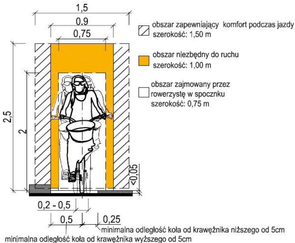
Rysunek 1. Skrajnia rowerowa
